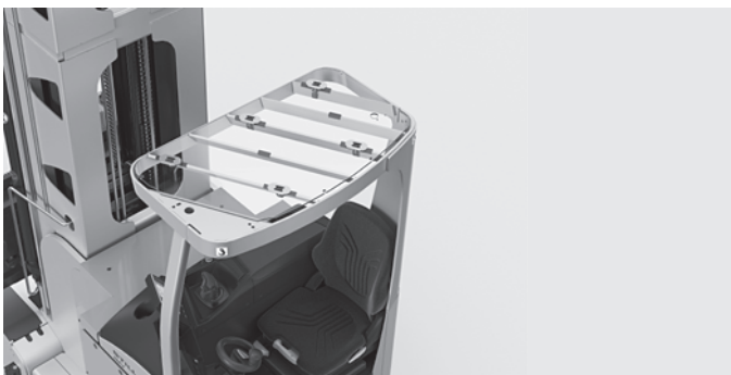
Quelle que soit l'application, nous proposons la protection de toit adéquate, à visibilité optimisée, avec ou sans couvercle en métal ou en polycarbonate
